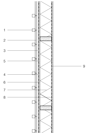
COUPE SUR FACADE RUE (VUE DE DESSUS) Mur rideau, bardage en frises à couvre-joints
