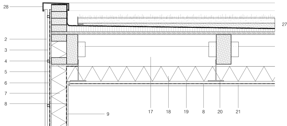
COUPE SUR TOITURE Toit terrasse végétalisé
